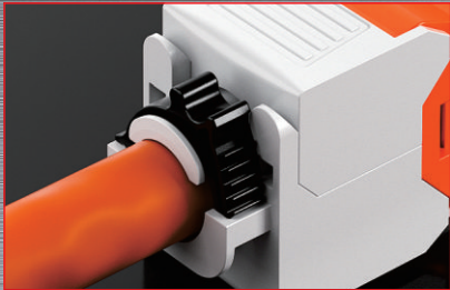
创新紧箍式六档锁扣结构设计无需扎带即可紧固
